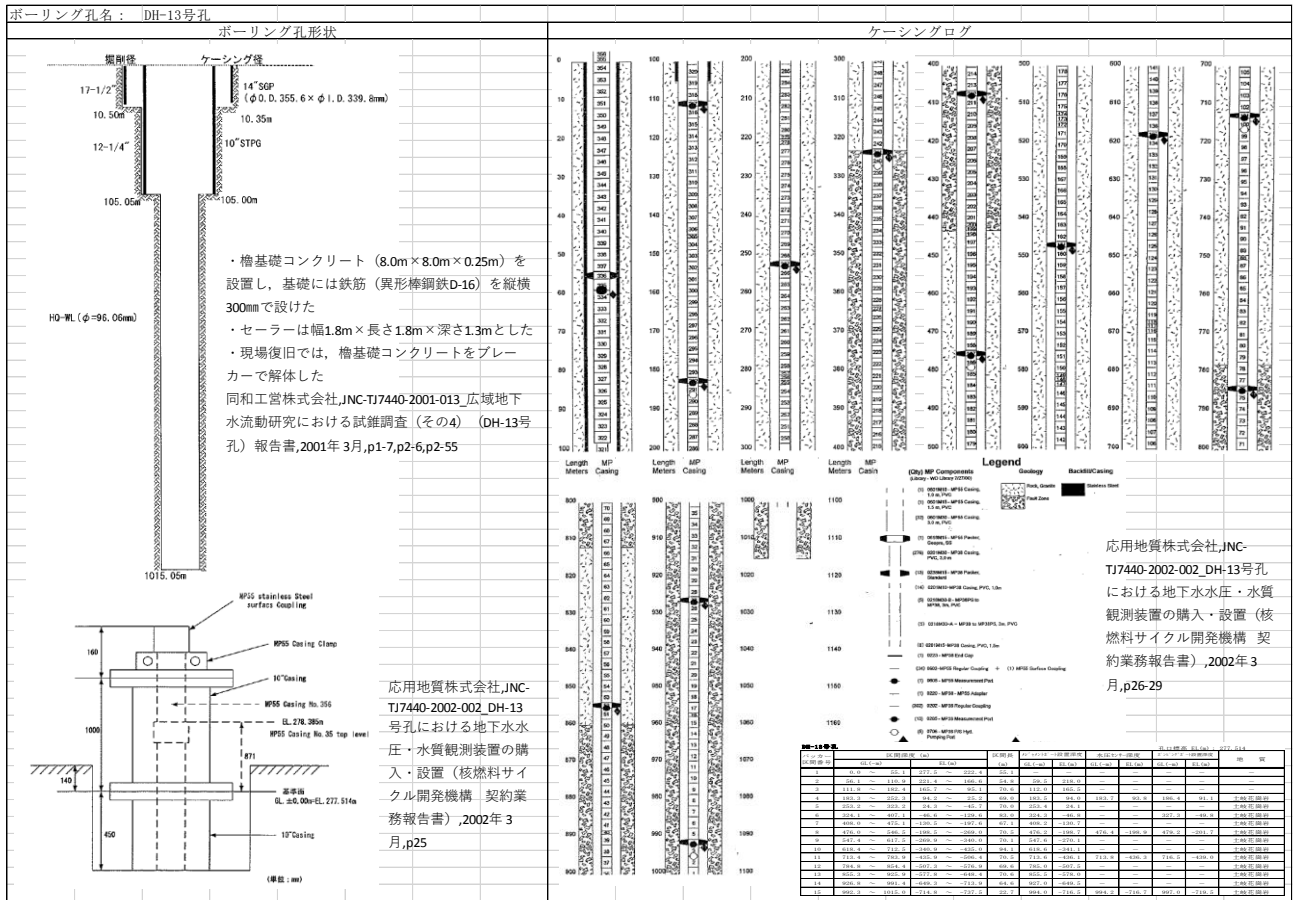
【別図 5.12】 各孔の現況 (DH-13)
