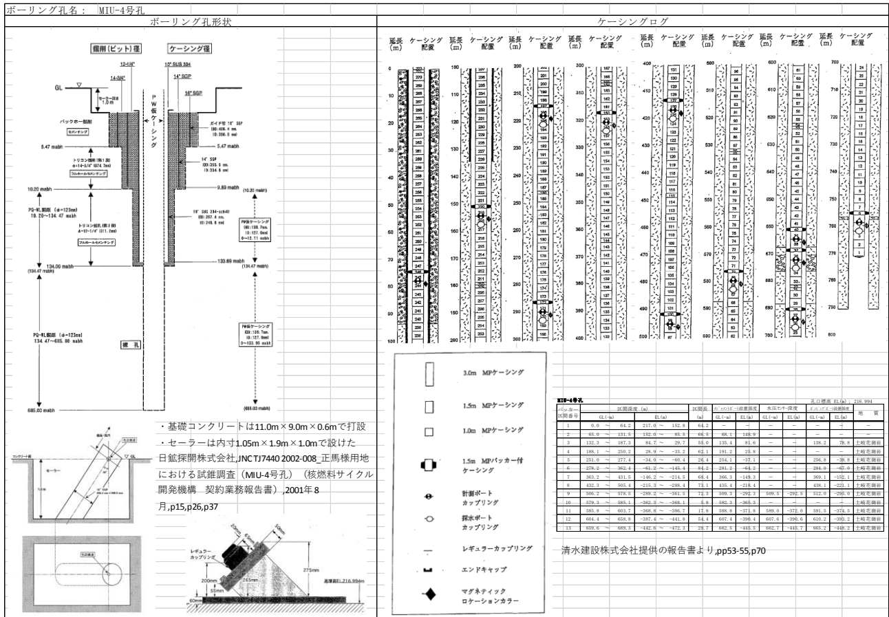
【別図 5.19】 各孔の現況 (MIU-4)
